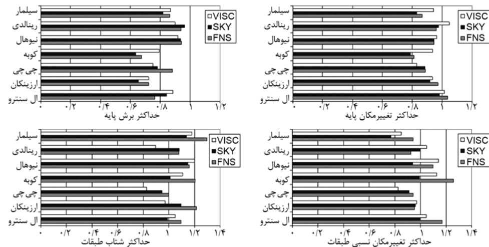
شکل ۱۱. شاخص‌های عملکرد، میرایی ویسکوز، الگوریتم اسکای- هوک و الگوریتم پیشنهادی FN-X , FN-Y .
