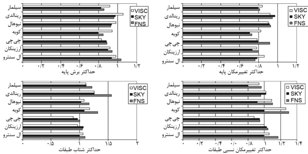
شکل ۱۰. شاخص‌های عملکرد، میرایی ویسکوز، الگوریتم اسکای- هوک و الگوریتم پیشنهادی FN-X , FN-Y .
