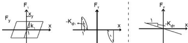
شکل 2. مؤلفه‌های F_1, F_{\dot{\gamma}} و F_{\dot{\gamma}} برای نیروی میرایی متغیر F_d در روش پیشنهادی.
